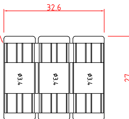
EFA04 71 P02 Ø3.4 COUPLER CLIP
